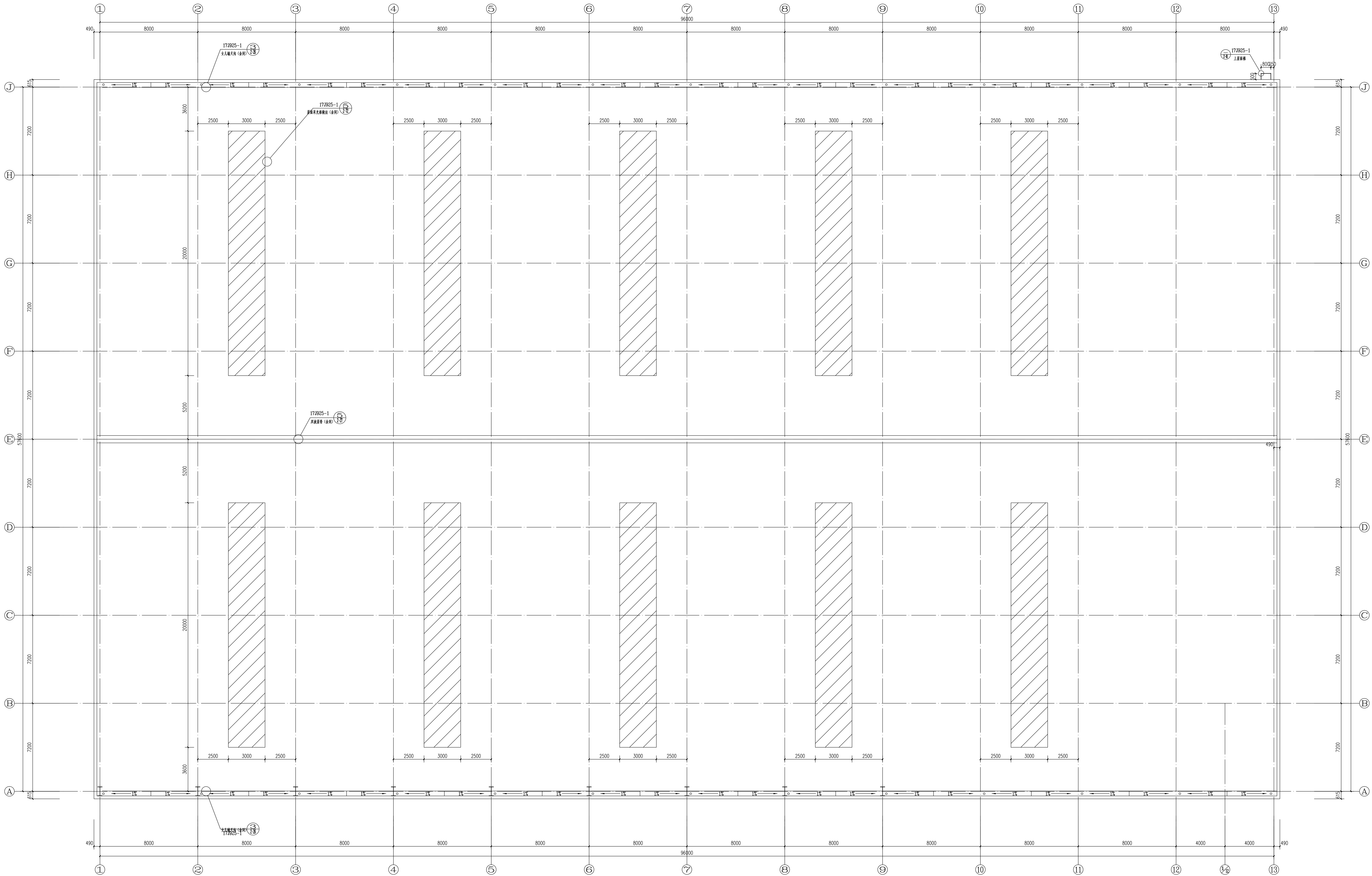
屋顶平面图 1:100
